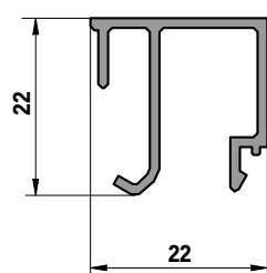
6225 (0,257 kg/m)
