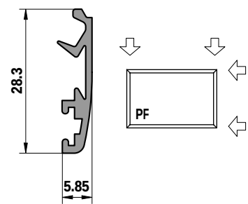
6206 (0,181 kg/m)
